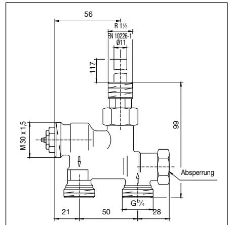
Tauchrohrventil Zweirohr mit senkrechter Lanze und Absperrung
